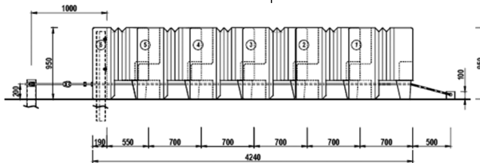
Schéma montáže – pohled z boku
