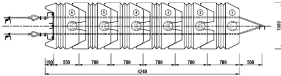
Schéma montáže – pohled ze shora
